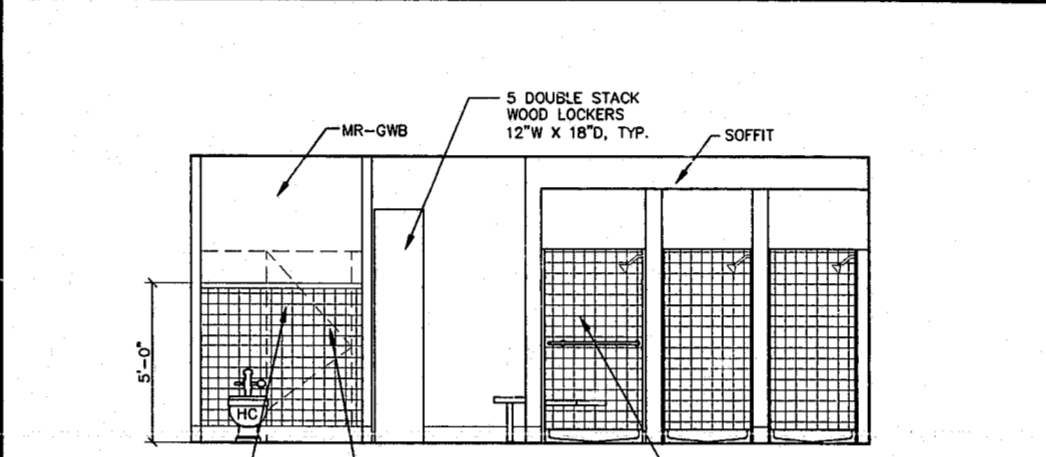
3 TOILET # 110 SCALE: 1/4" = 1'-0"
