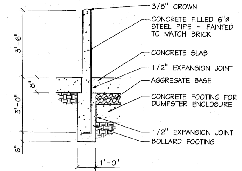
3 TRASH ENCLOSURE BOLLARD SCALE: 1/2" = 1'-0"
