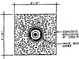
5 2" BLOW-OFF ASSEMBLY 12 N.T.S.
