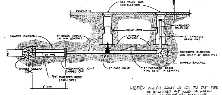
5 2" BLOW-OFF ASSEMBLY 12 N.T.S.
