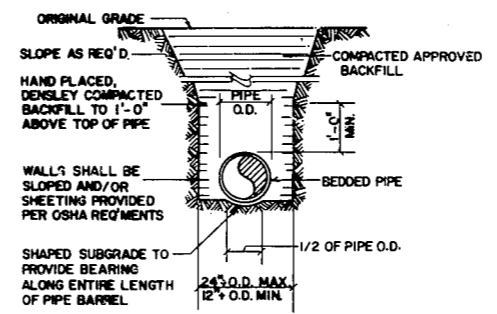
9 PIPE LAYING CONDITION 12 N.T.S.
