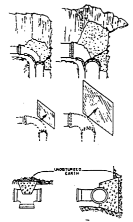
2 THRUST BLOCKING 12 N.T.S.
