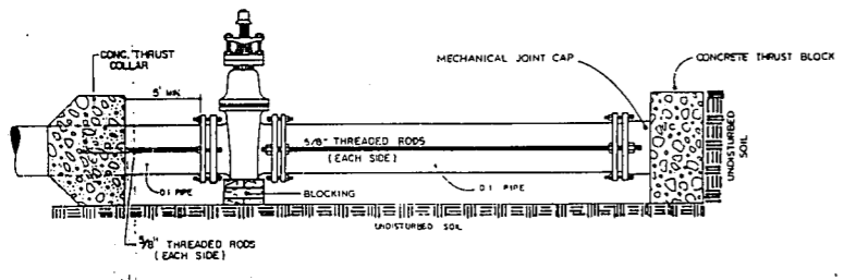
3 CAPPING DETAIL 12 N.T.S.
