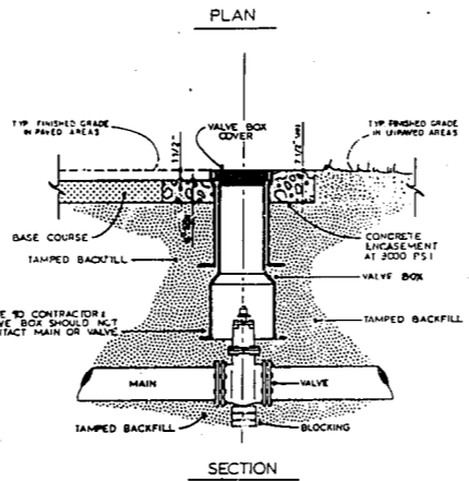
6 VALVE BOX INSTALLATION 12 N.T.S.
