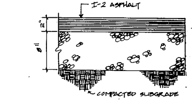
21 HEAVY-DUTY PAVING L-5 N.T.S.
