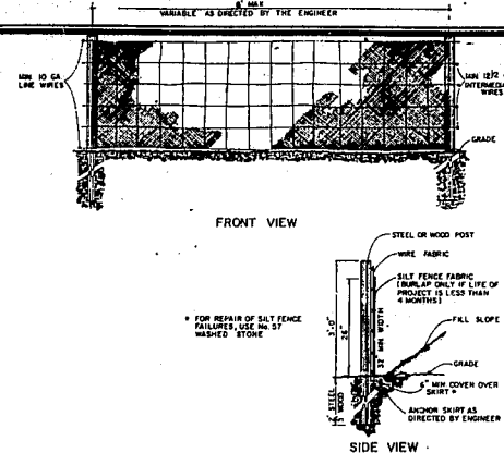
15 SILT FENCE L-5 N.T.S.
